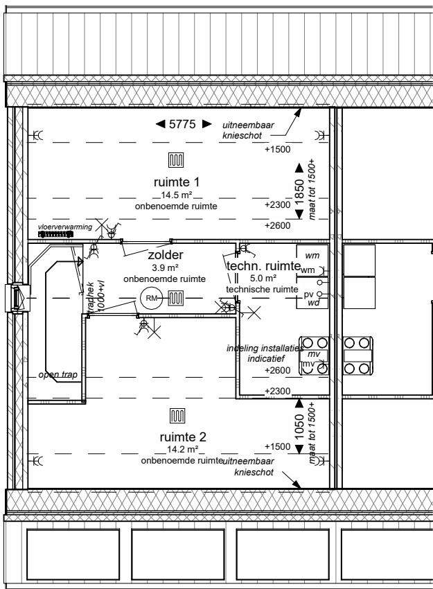
Tweede verdieping - Optie indeling
