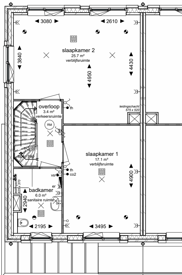
Eerste verdieping - Slaapkamers 2 en 3 samenvoegen optie 1
