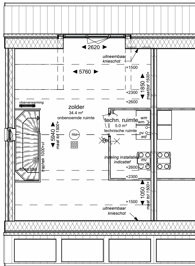
Tweede verdieping - Optie Dakkapel
