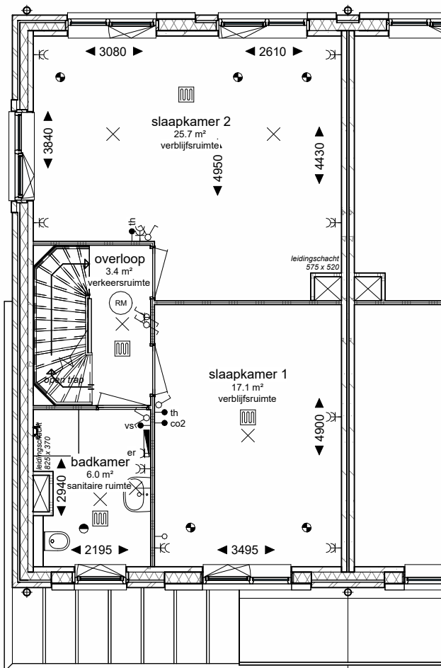
Eerste verdieping - Slaapkamers 2 en 3 samenvoegen optie 2
