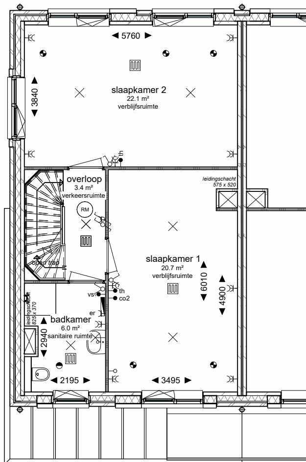
Eerste verdieping - Slaapkamers 2 en 3 samenvoegen optie 3
