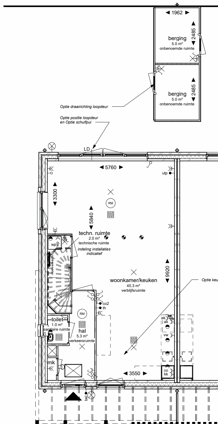
Begane grond - Optie
