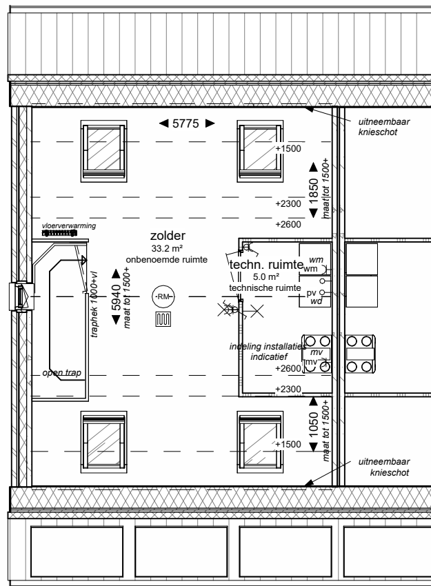
Tweede verdieping - Optie dakraam
