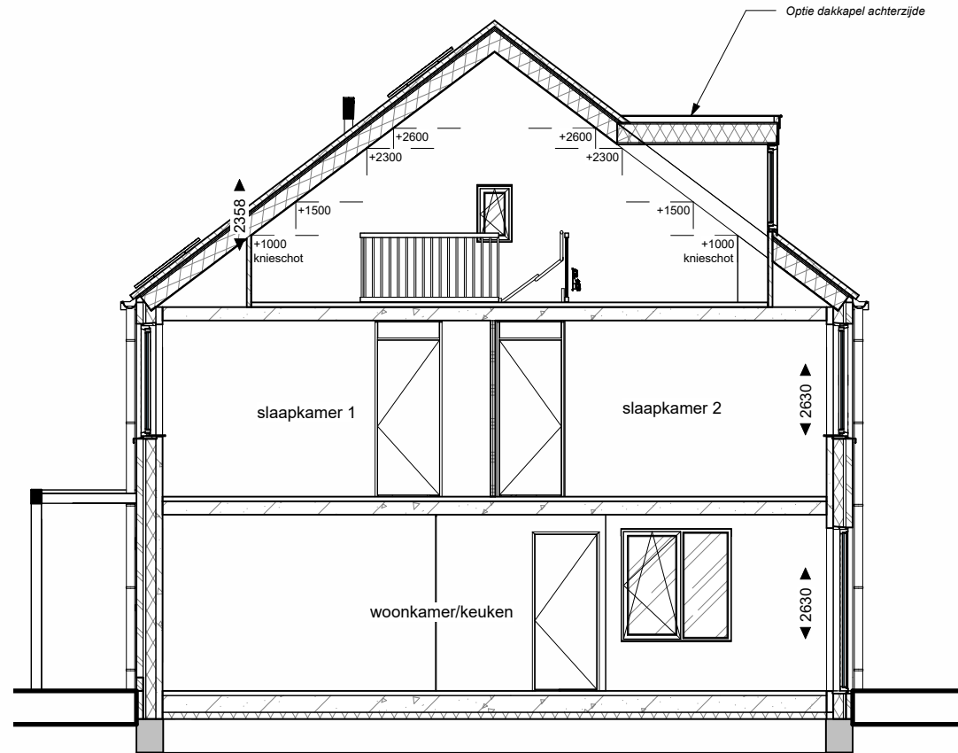
Doorsnede A - Optie dakkapel
