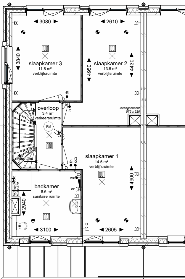
Eerste verdieping - Optie vergroten Badkamer
